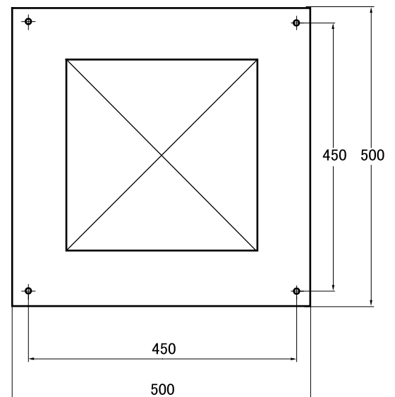
ベース寸法図 上方より
